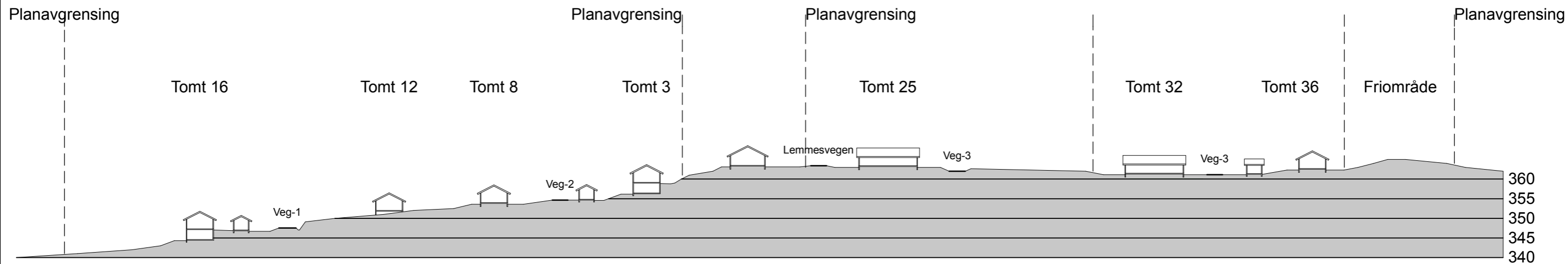
Terrengsnitt 1
